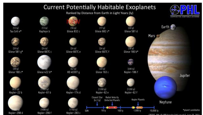
Cuerpos espaciales que forman parte del catálogos de exoplanetas.
